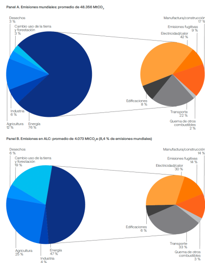
Gráfico 1.3 Emisiones de GEI por sector para el período 2015-2019 Fuente: Elaboración propia con base en datos de Climate Watch (s.f).
